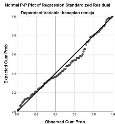
Gambar 1. Plot P-P Normal Dari Residual Standar Regresi
